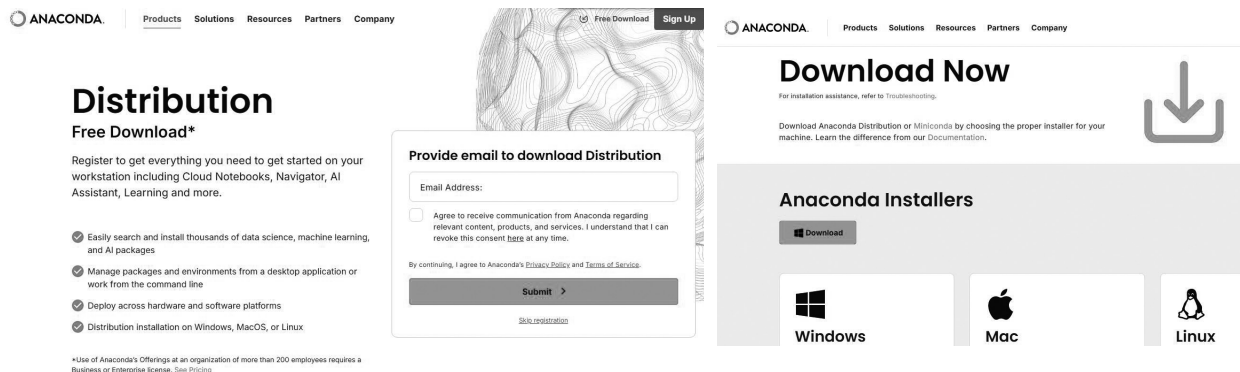
图 1-7 选择版本
