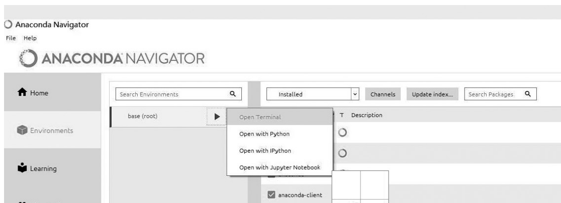
图 1-11 运行终端
