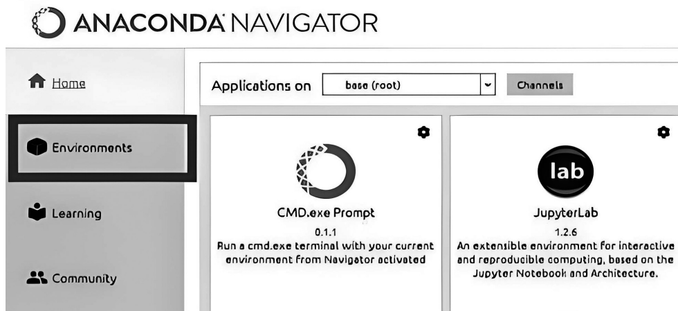
图 1-10 点击 Environment
